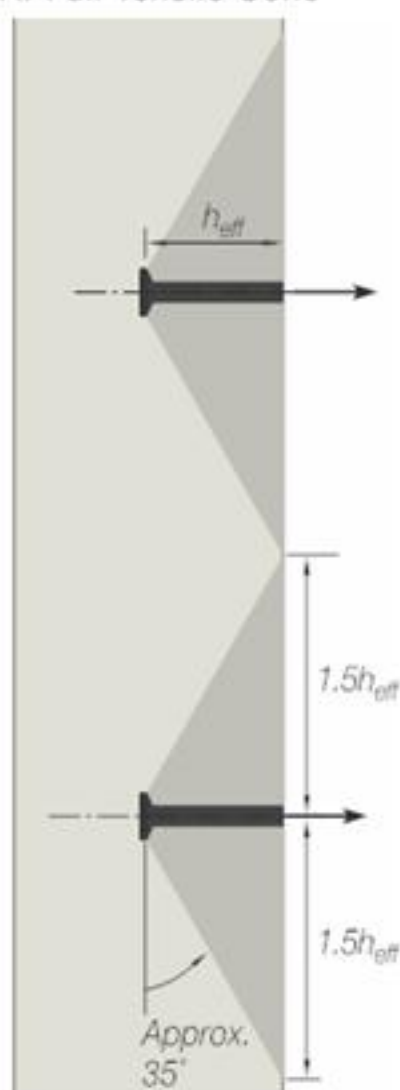
Fig A. Full Tensile Cone
